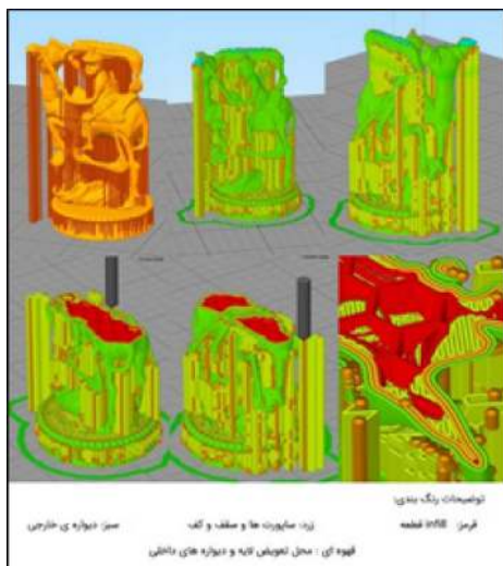
■ شکل ۱۸: ساپورت‌گذاری در نرم‌افزار Simplify3D (مأخذ: نگارندگان).
